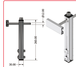
ALUMINIUM HOLDER 30X30 + PROFIL
